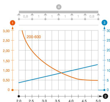
Диаграма на натоварване за кабелна стълба тип LG 110 VS
